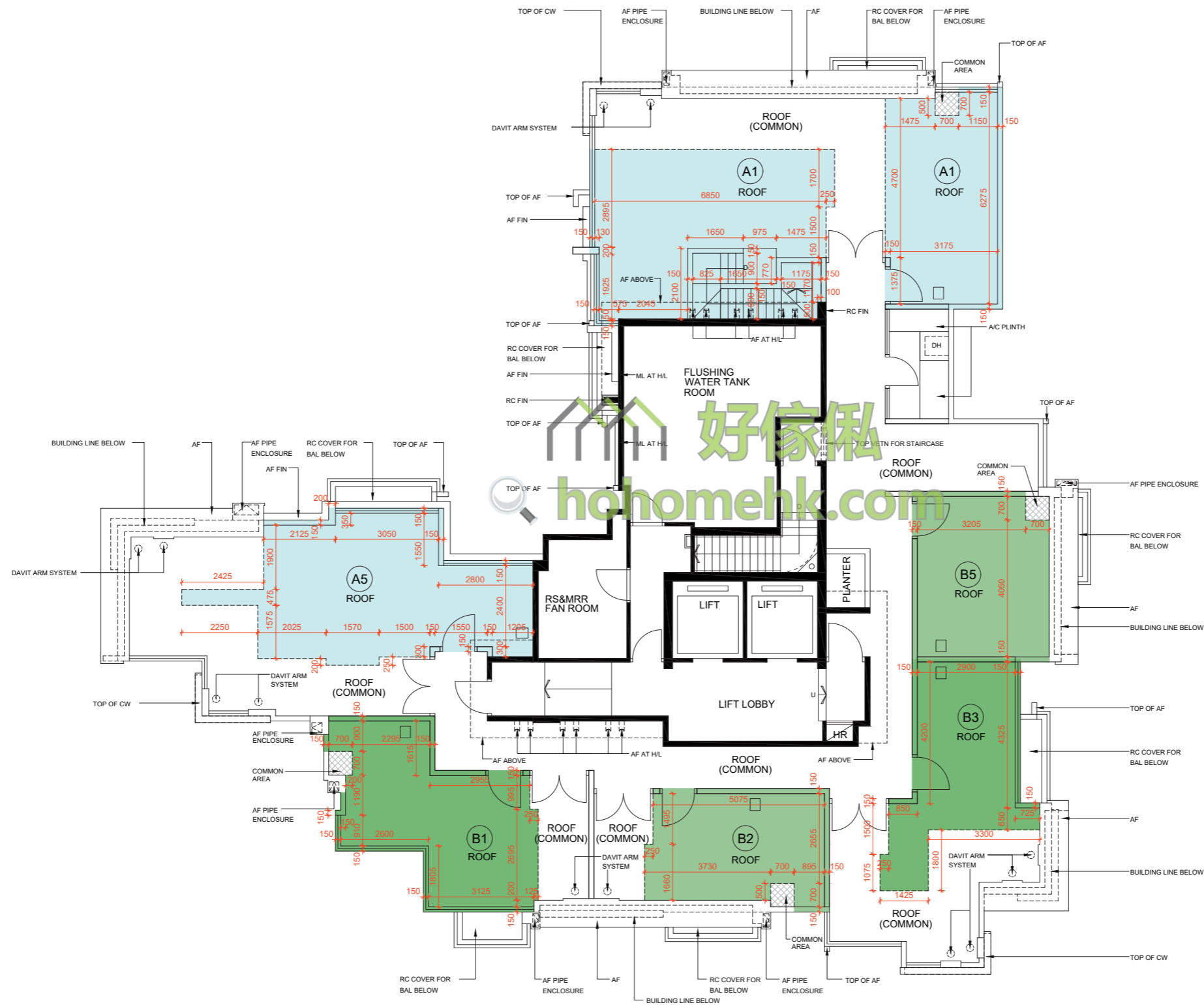
SCENIC TOWER 6 ROOF FLOOR PLAN 優景閣第6座 天台平面圖
