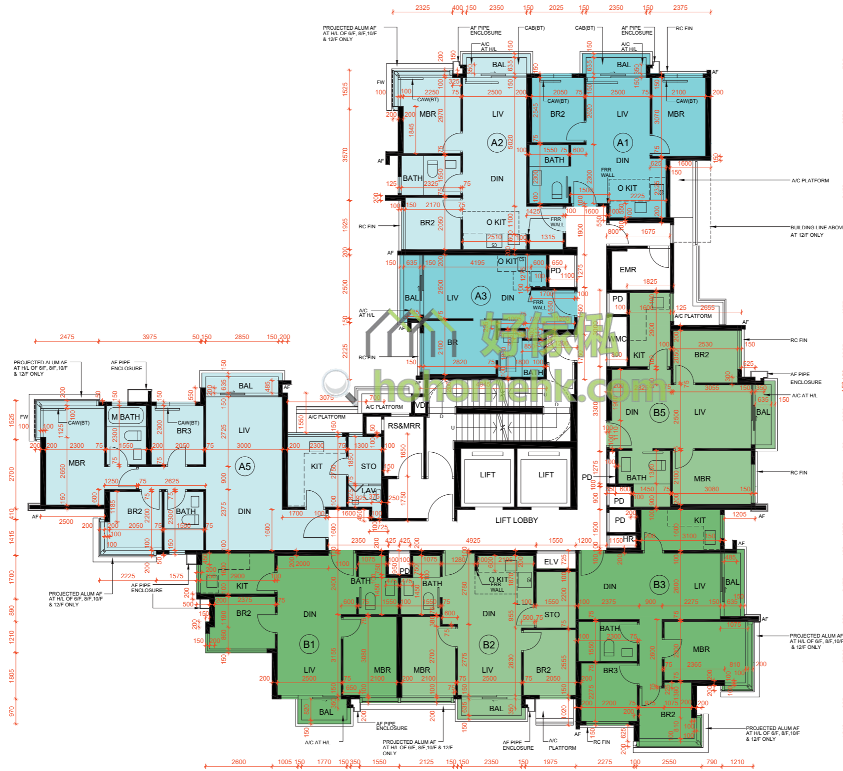
SCENIC TOWER 6 5/F-12/F FLOOR PLAN 優景閣第6座 5樓至12樓平面圖
