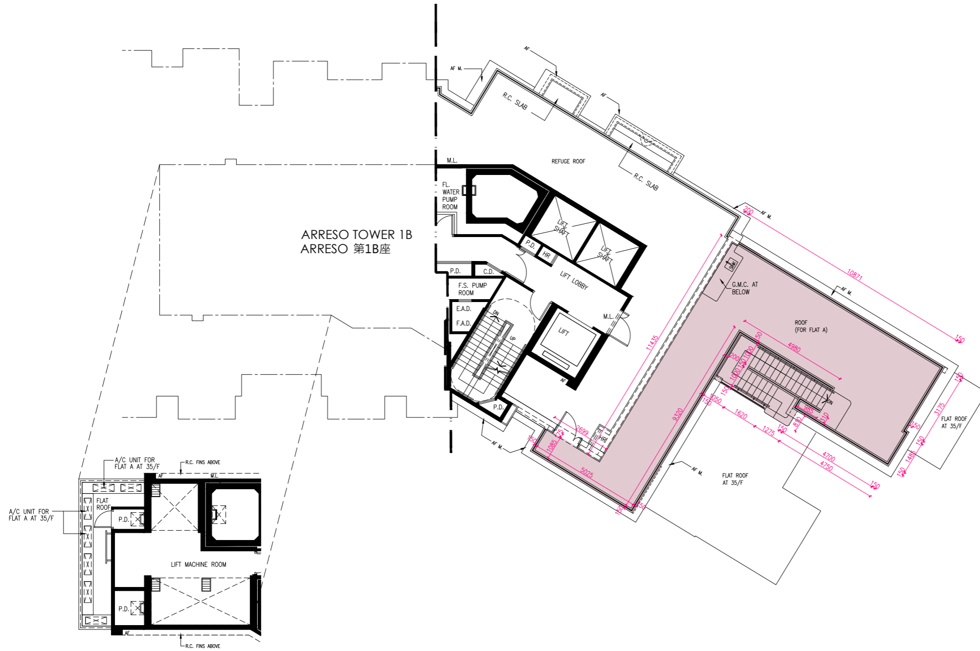
PART PLAN OF UPPER ROOF 上層天台部分平面圖
