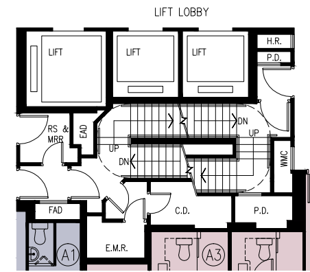
PART PLAN OF 32/F 32樓部分平面圖
