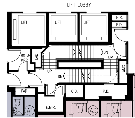
PART PLAN OF 33/F 33樓部分平面圖
