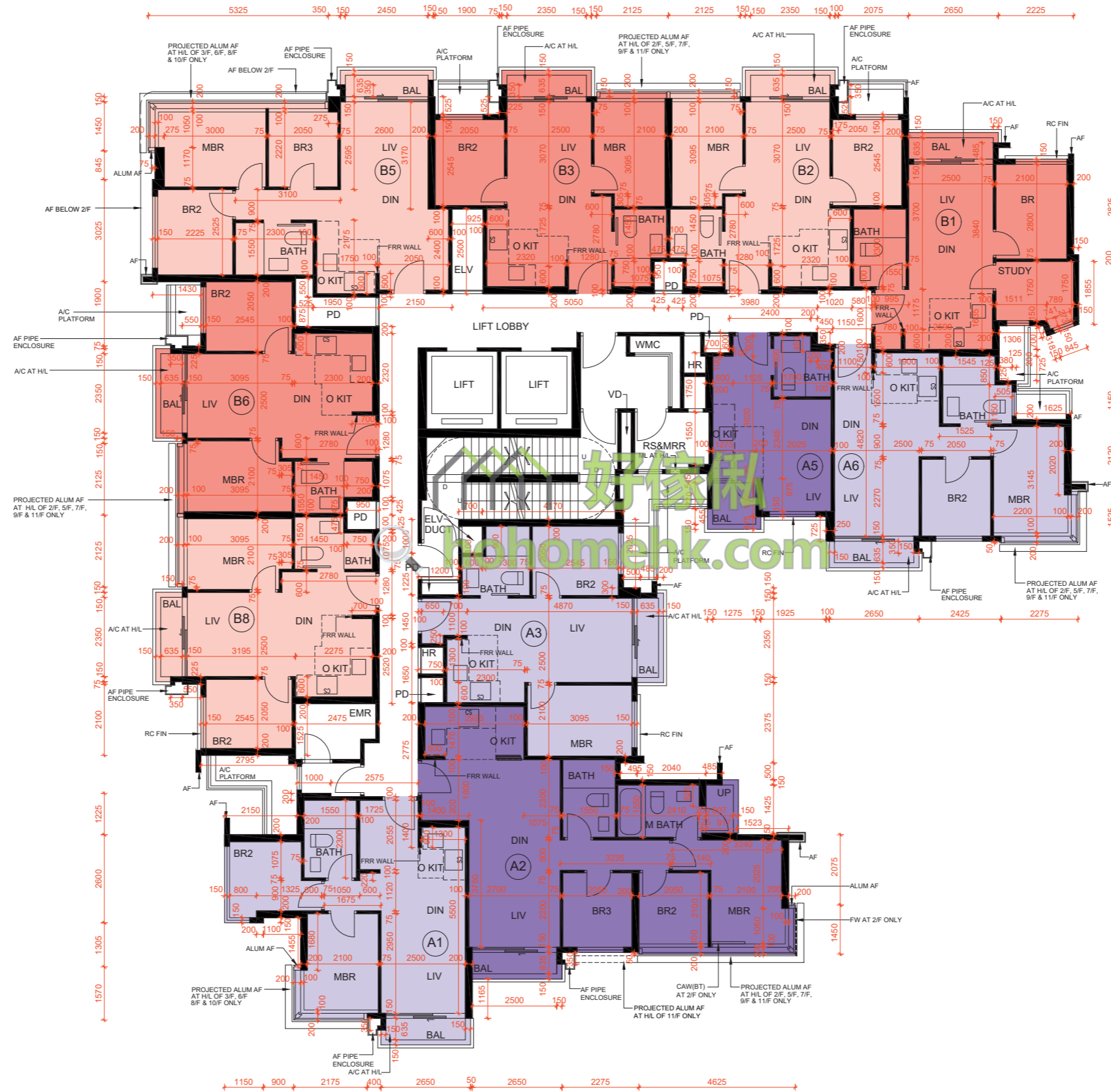
GREENWOOD TOWER 5 2/F-3/F AND 5/F-11/F FLOOR PLAN 翠景閣第5座 2樓至3樓 及 5樓至11樓平面圖
