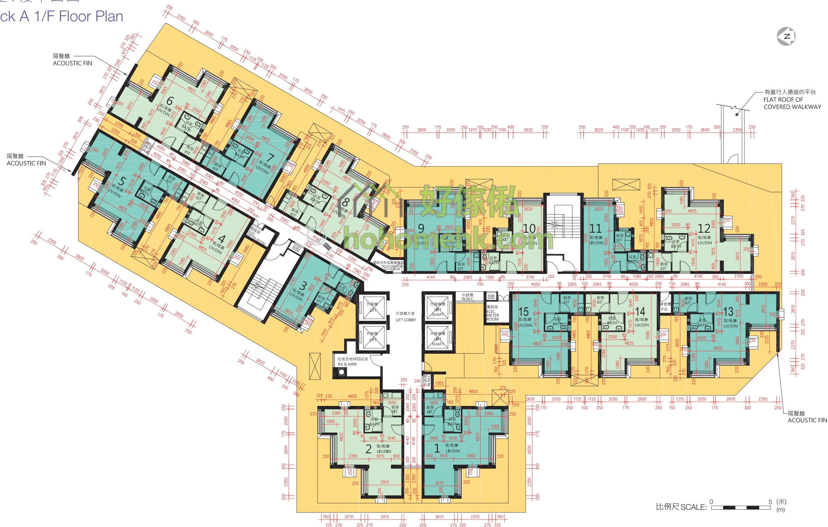
A 座1樓平面圖
